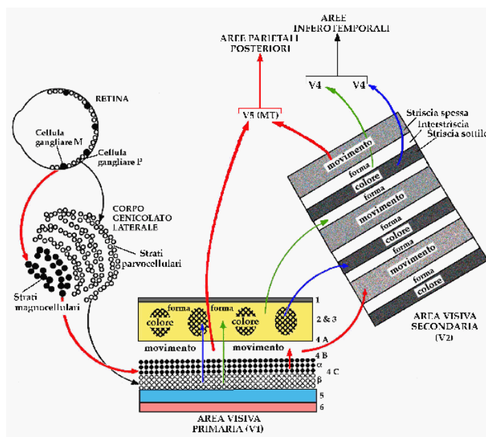
Fig. 25/1. Rappresentazione schematica della distribuzione dei canali magnocellulare e parvocellulare dalla retina alle aree parietali posteriori ed inferotemporali, attraverso il corpo genicolato laterale e le aree visive V1 e V2. Modificata da Livingstone e Hubel, 1988.
